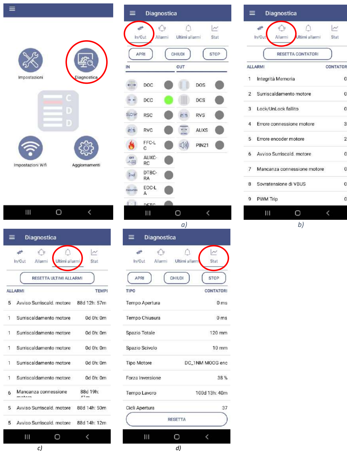
Figura 10 - (a) Ingressi/Uscite (b) Lista contatori allarmi (c) Lista ultimi allarmi ordinati dal più recente al meno recente (d) Statistiche
