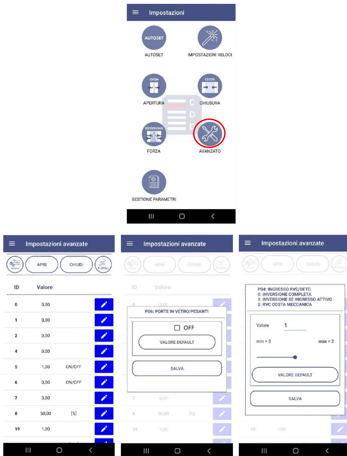
Fig. 15 - (a) Lista dei parametri; (b) Impostazione valore binario; (c) Impostazione valore con range
