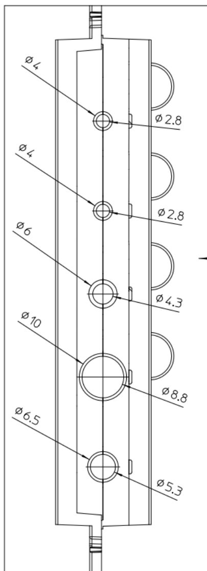
Figura 3: Motorseite
