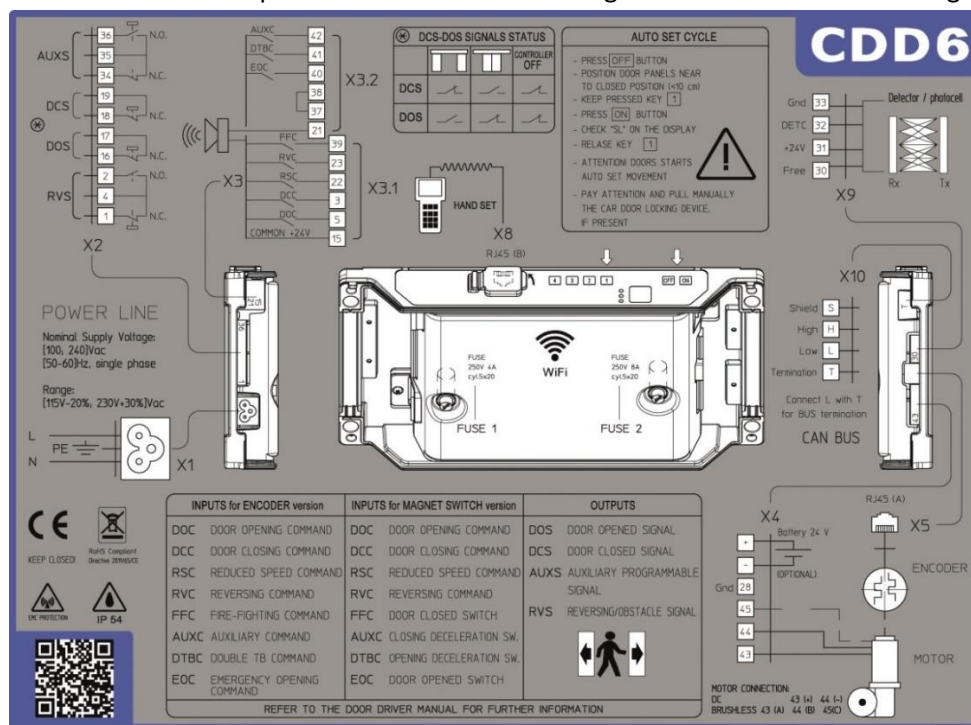
- Abbildung 2-1: Anschlussübersicht CDD6
