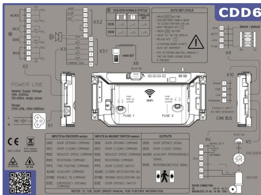
- Abbildung 4-1: Anschlussschaltplan CDD6 -
