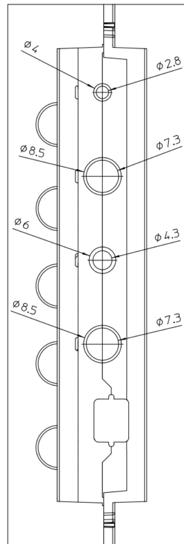
Figura 4: Einspeiseseite
